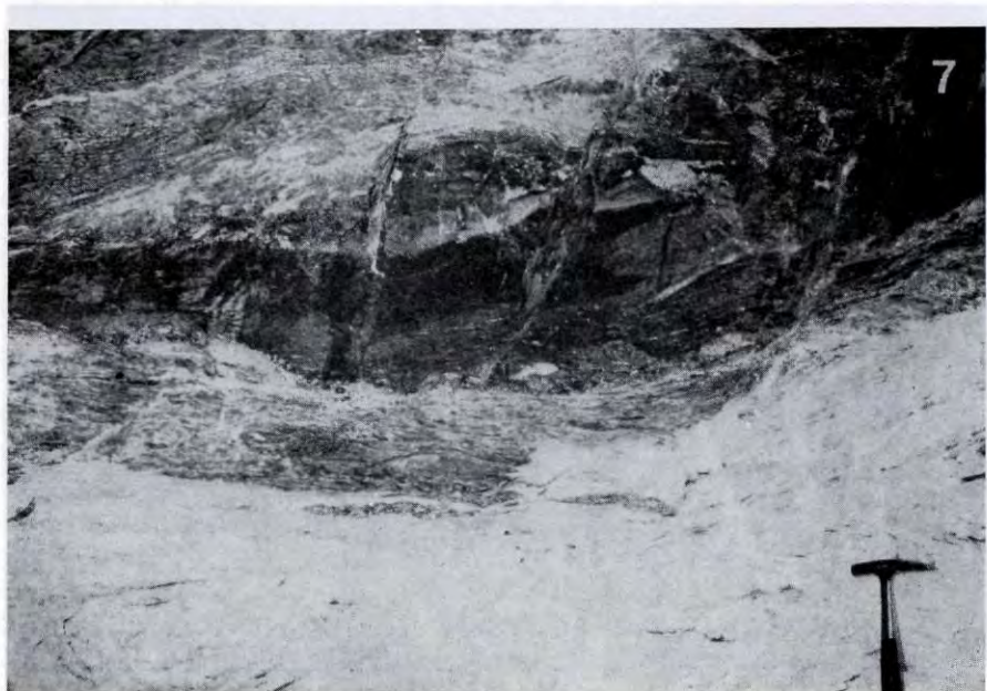
7. Lente di scisto ovarditico (scuro) nel talco frammisto a clorite e passante a mica-cloritescisto; in basso, talco bianco
