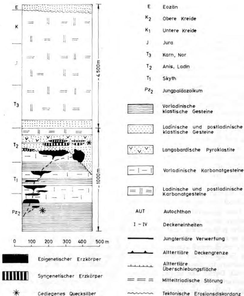
Abb. 1. Schematisches Säulenprofil durch das Idrija Gebiet
